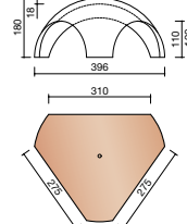
P000 5730 Jonction 1 faitière 255 mm et 2 arêtiers 210 mm
