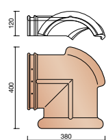
P000 5120 Rencontre 2 faitières 230 mm et 1 arêtier 190 mm
