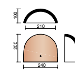
P000 3360 About d'arêtier demi-rond sans emboîtement 210 mm
