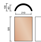
P000 3300 Arêtier demi-rond sans emboîtement 210 mm (3,1 au ml)
