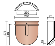
P000 1260 About d'arêtier demi-rond 230 mm
