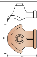
P000 5290 Rencontre porte-boule 1 faitière 230 mm et 2 arêtiers 190 mm (+ 5900 ou 5950)
