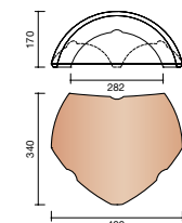
P000 5500 Jonction 1 faitière 230 mm et 2 arêtiers 230 mm
