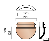
P000 3110 About d'arêtier demi-rond à emboîtement 190 mm
