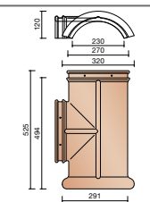
P000 5020 Rencontre 3 faitières 230 mm
