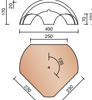
P000 5740 Jonction 1 faitière 230 mm et 2 arêtiers 190 mm
