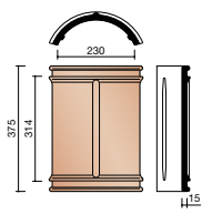
P000 1230 Faitière demi-ronde à double emboîtement 230 mm
