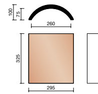
P000 1400 Faitière demi-ronde sans emboîtement 255 mm (3,1 au ml)
