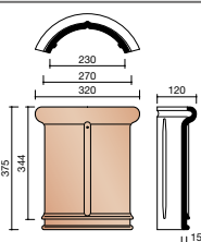
P000 1200 Faitière demi-ronde 230 mm (3,0 au ml)
