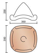
P000 5630 Rencontre 4 arêtiers 190 mm sans porte-boule
