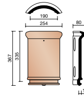
P000 3100 Arêtier demi-rond à emboîtement 190 mm (3,0 au ml)
