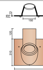
ETEM 8770 Tuile à douille Ø 160 mm (176 cm 2 )
