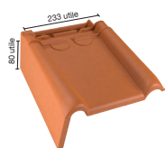
BOPA 7080 Tuile à rabat G (3,9 au ml)
