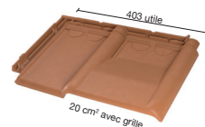
BOPA 8640 Tuile chatière (20 cm 2 ) (0,10 pc / m 2 projeté) ♦
