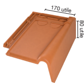
BOPA 7090 Tuile à rabat D (3,9 au ml)
