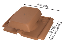
BOPA 8729 Kit tuile à douille Ø 150 mm (165 cm 2 ) (Conforme DTU et RE 2020 VMC)
