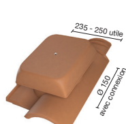
MK10 8729 Kit tuile à douille Ø 150 mm (165 cm 2 ) + Ventex (conforme DTU 68.3)
