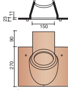
EGAYR 8770 Tuile à douille Ø 160 mm (176 cm 2 ) (Conforme au DTU et RE 2020 VMC)
