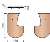
EGAYE 8680 Paire de tuiles sous-chatière écaille
