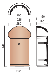
E000 1160 About arêtier 1/2 rond à emboîtement
