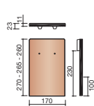
EGAYR 0000 Tuile rectangulaire
