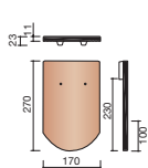
EGAYE 0000 Tuile écaille
