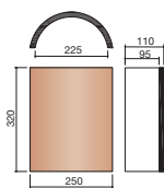
E000 1400 Faîtière 1/2 ronde sans emboîtement (3,1 au ml)
