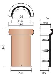
E000 1100 Faîtière 1/2 ronde à emboîtement (2,5 au ml)
