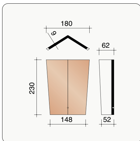
P0003701 6 pièces/m crt Cornier
