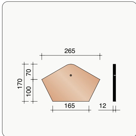
P0002841 Fronton pour faîtière angulaire sans emboîtement 30°
