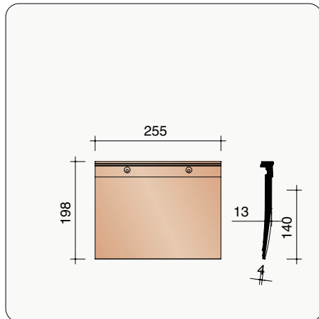
PELF8110 4 pièces/m crt Tuile raccourcie
