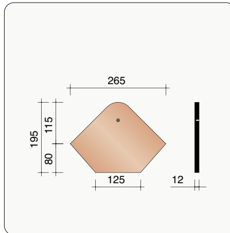
P0002842 Fronton pour faîtière angulaire sans emboîtement 45°
