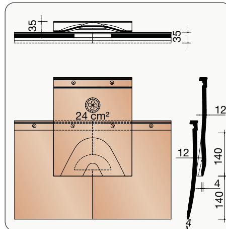
PELF8611 Kit de ventilation avec grille - 24 cm²
