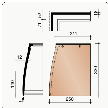
PELF8800 3,6 pièces/m crt Pièce d'angle gauche bardage (collée)
