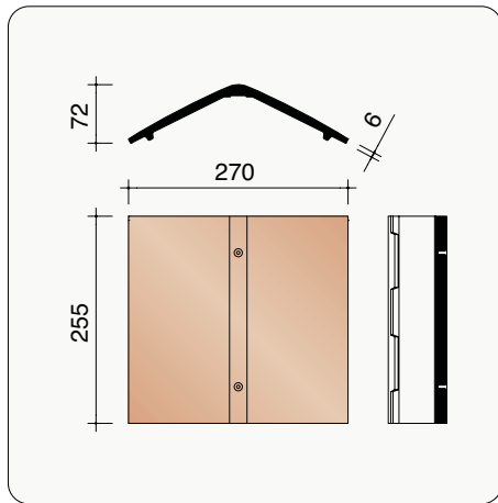
P0002801 4 pièces/m crt Faîtière angulaire sans emboîtement 30°
