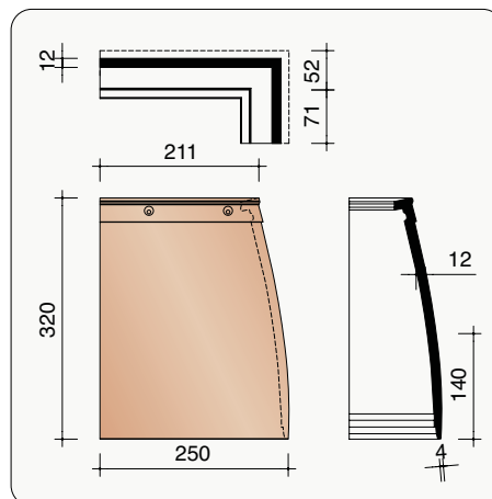
PELF8810 3,6 pièces/m crt Pièce d'angle droite bardage (collée)
