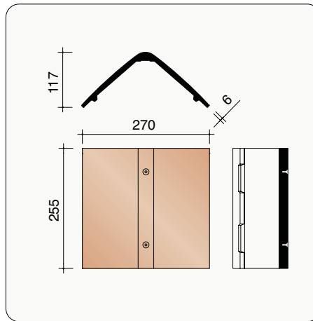
P0002802 4 pièces/m crt Faîtière angulaire sans emboîtement 45°
